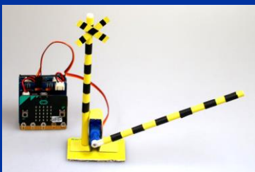
センサー付き遮断器
